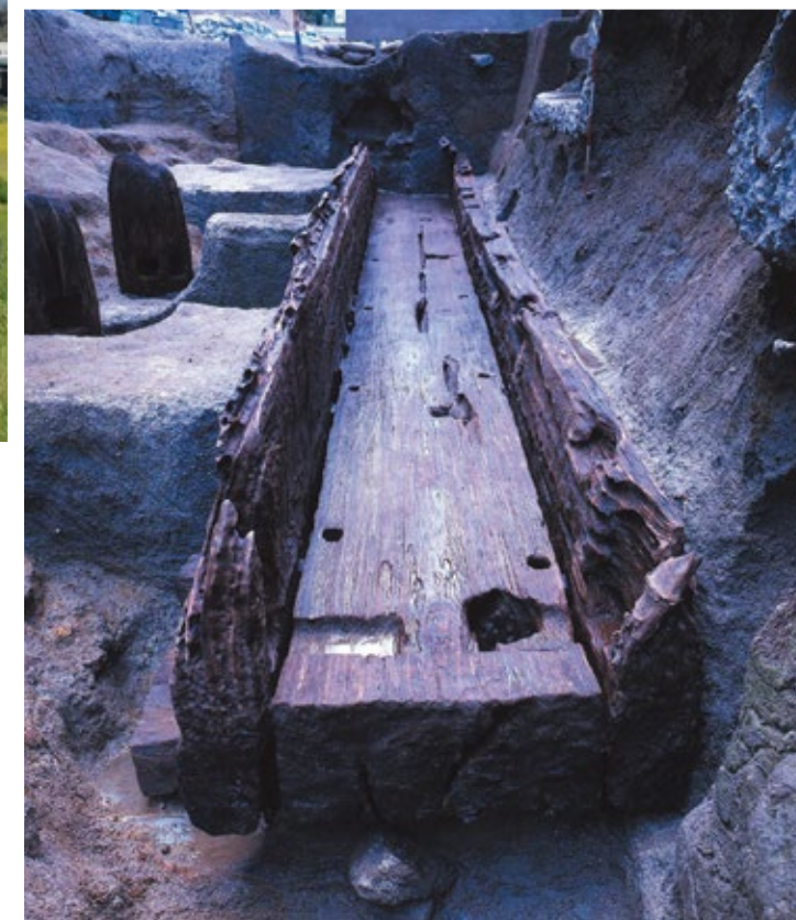
木制导水管
